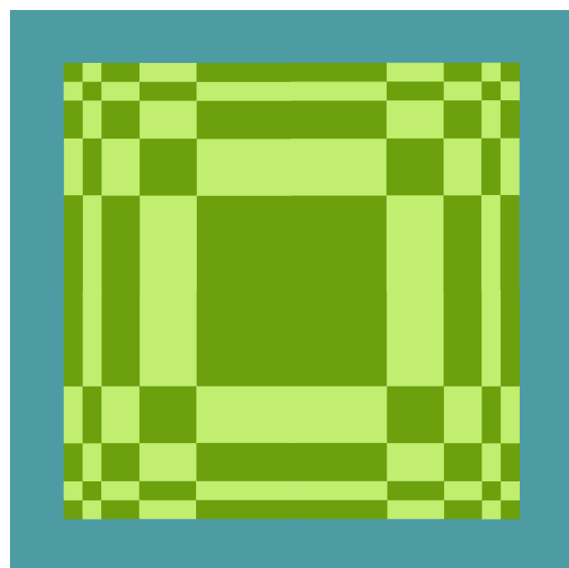
Abbildung 4: Fibonacci-Muster
