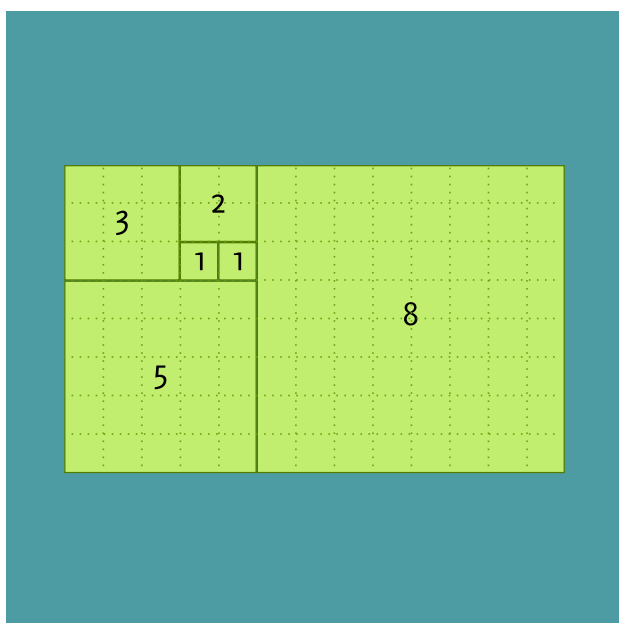
Abbildung 3: Fibonacci-Folge
