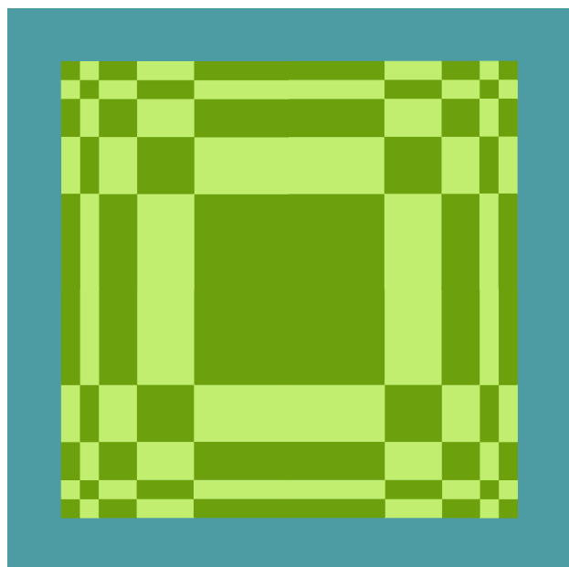
Abbildung 4: Fibonacci-Muster
