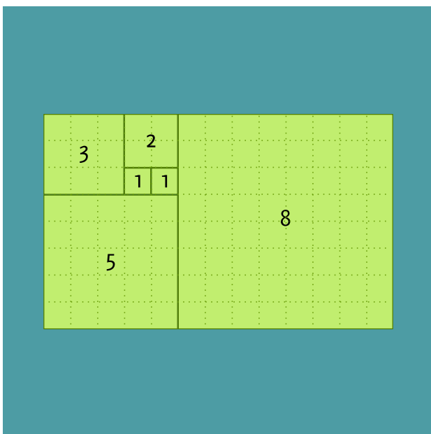
Abbildung 3: Fibonacci-Folge
