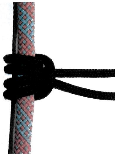
Abbildung 12: Prusikknoten [1]
